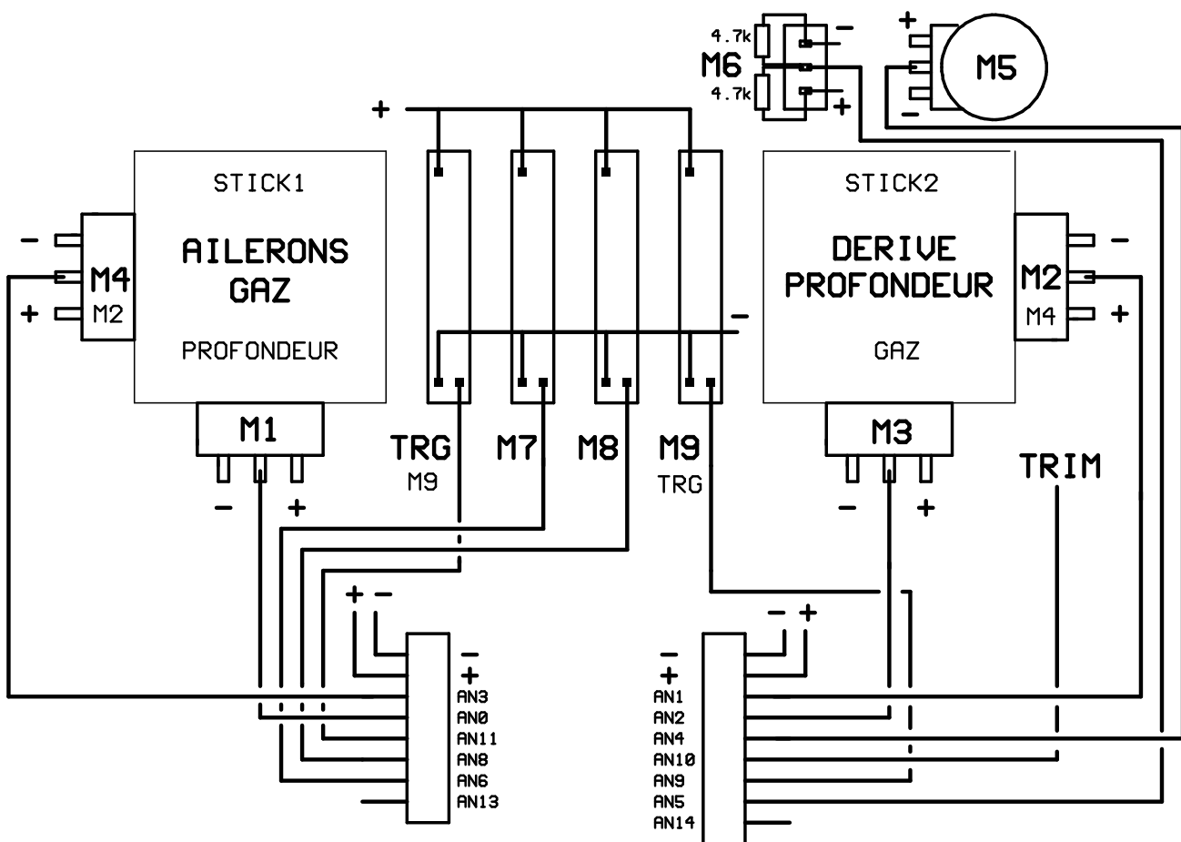
CONNEXION des ACTIONNEURS
